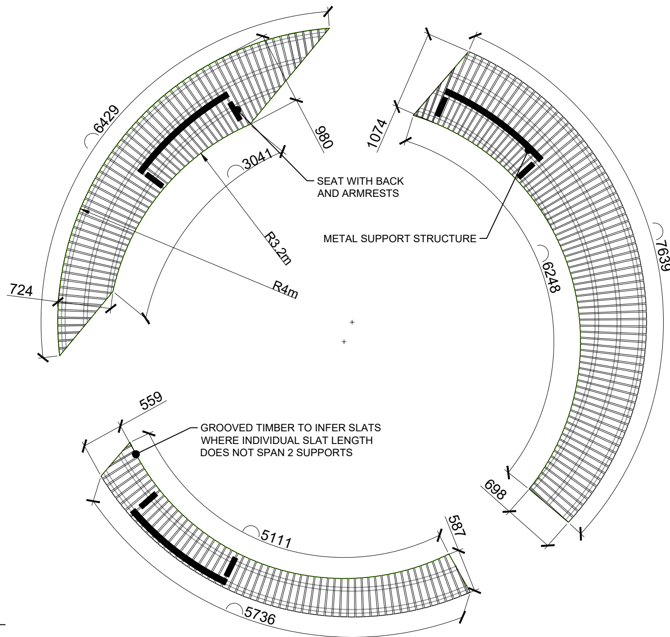
3 PLAN 1:50
