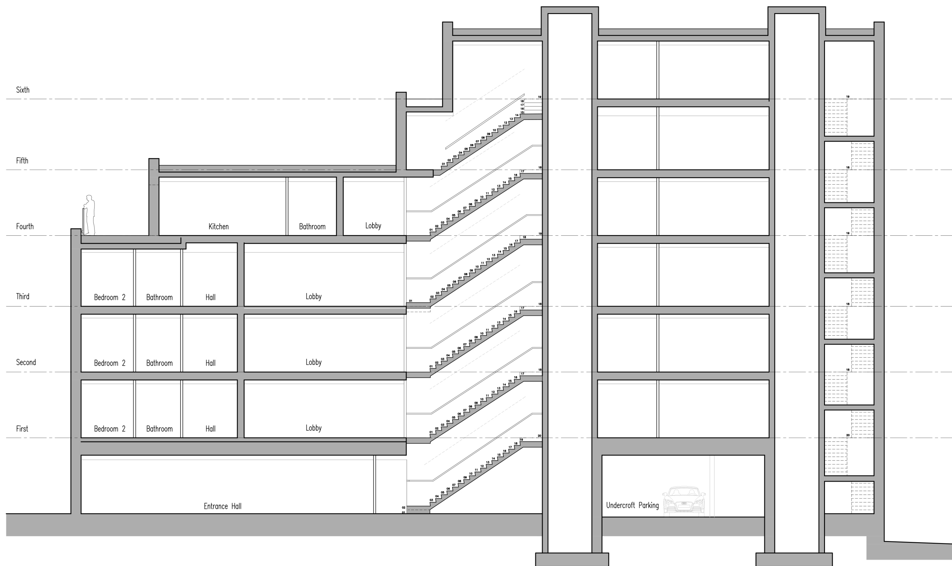
Section A-A
