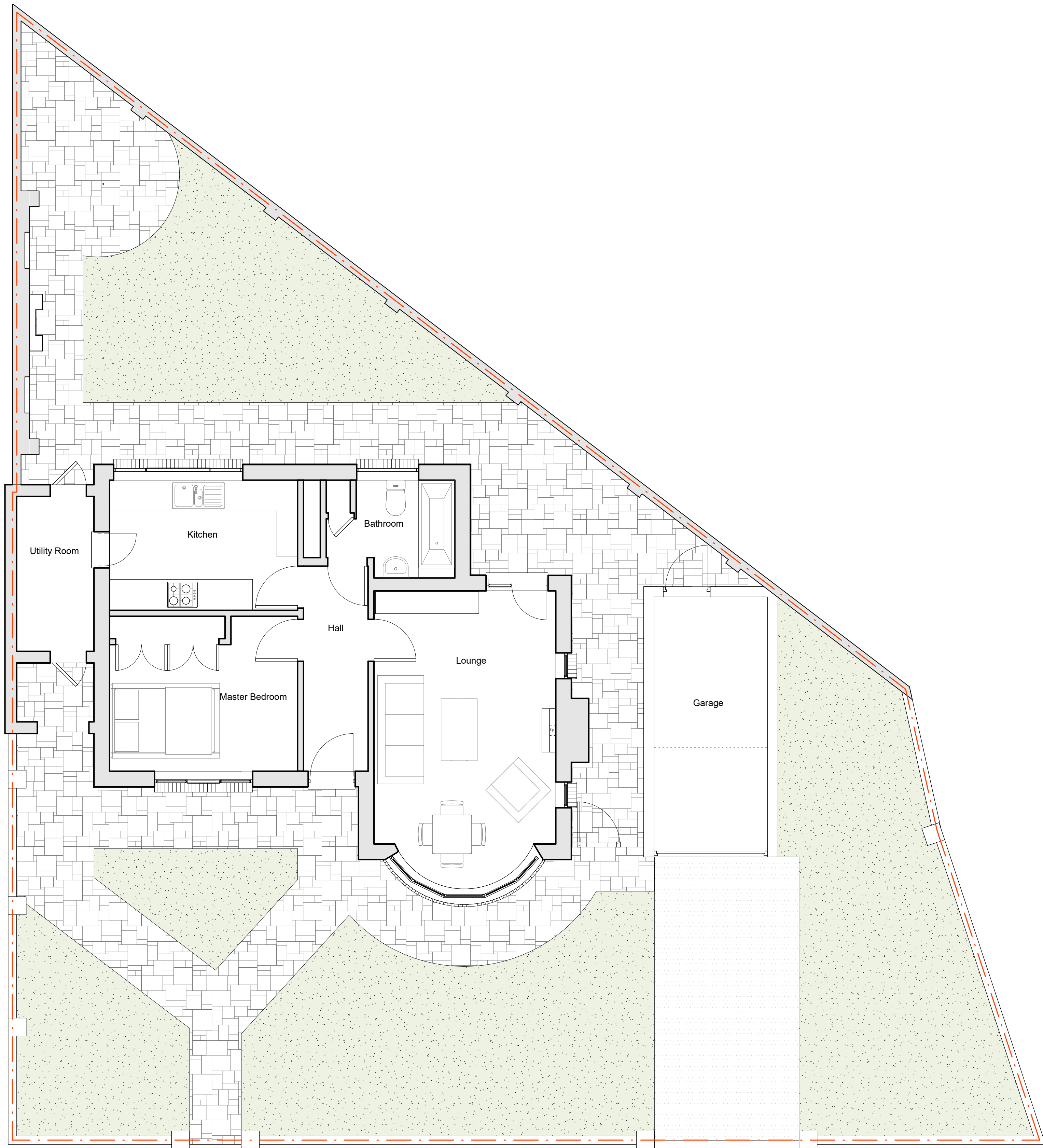
1 EXISTING GF 2000 Scale: 1 : 50
