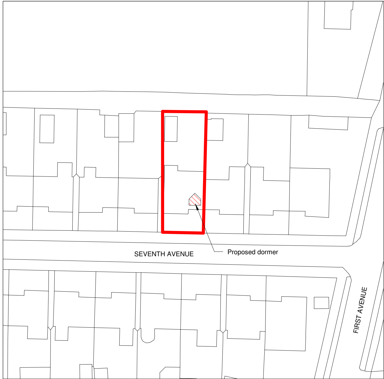
1 SITE PLAN 1 : 500
