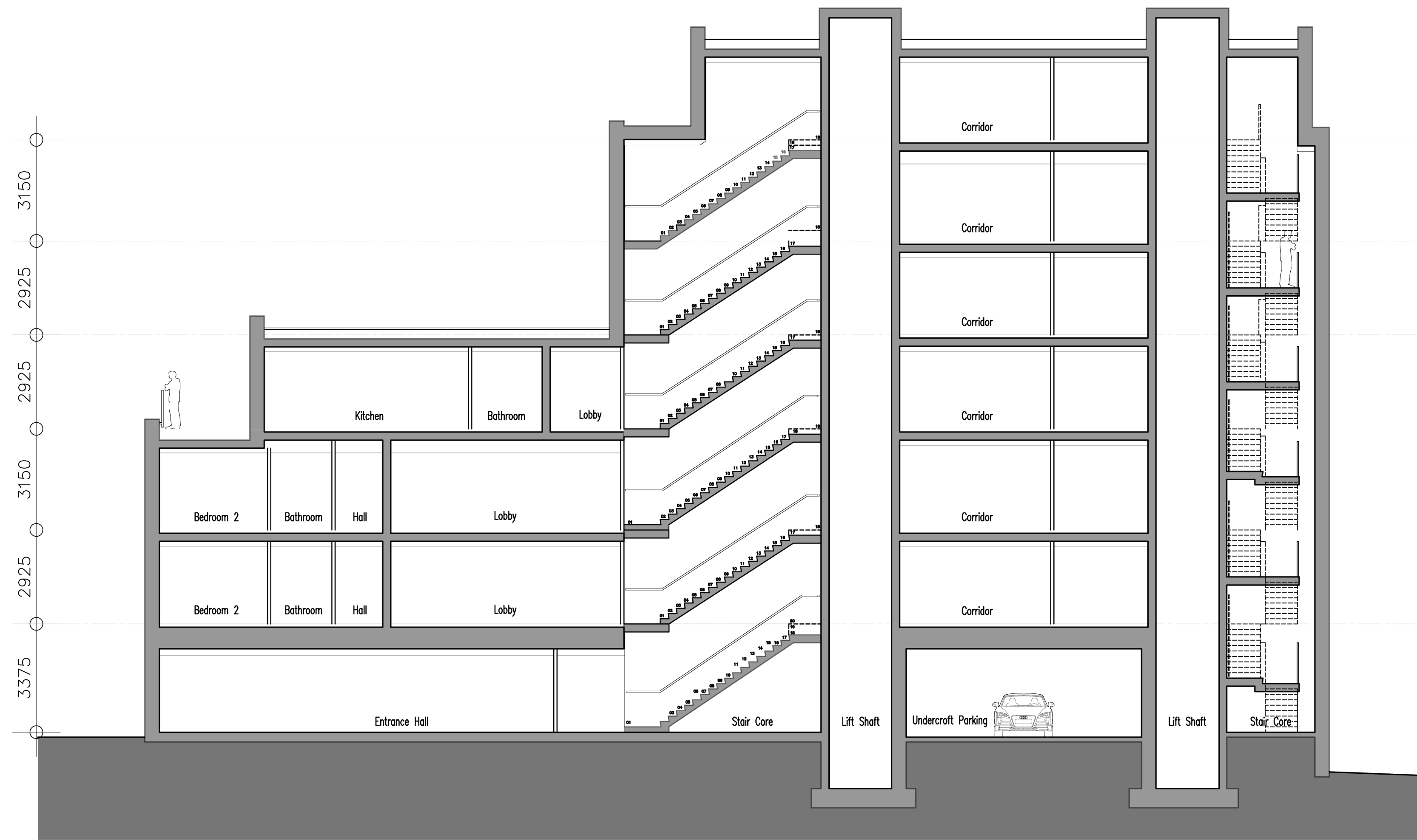
Section A-A
