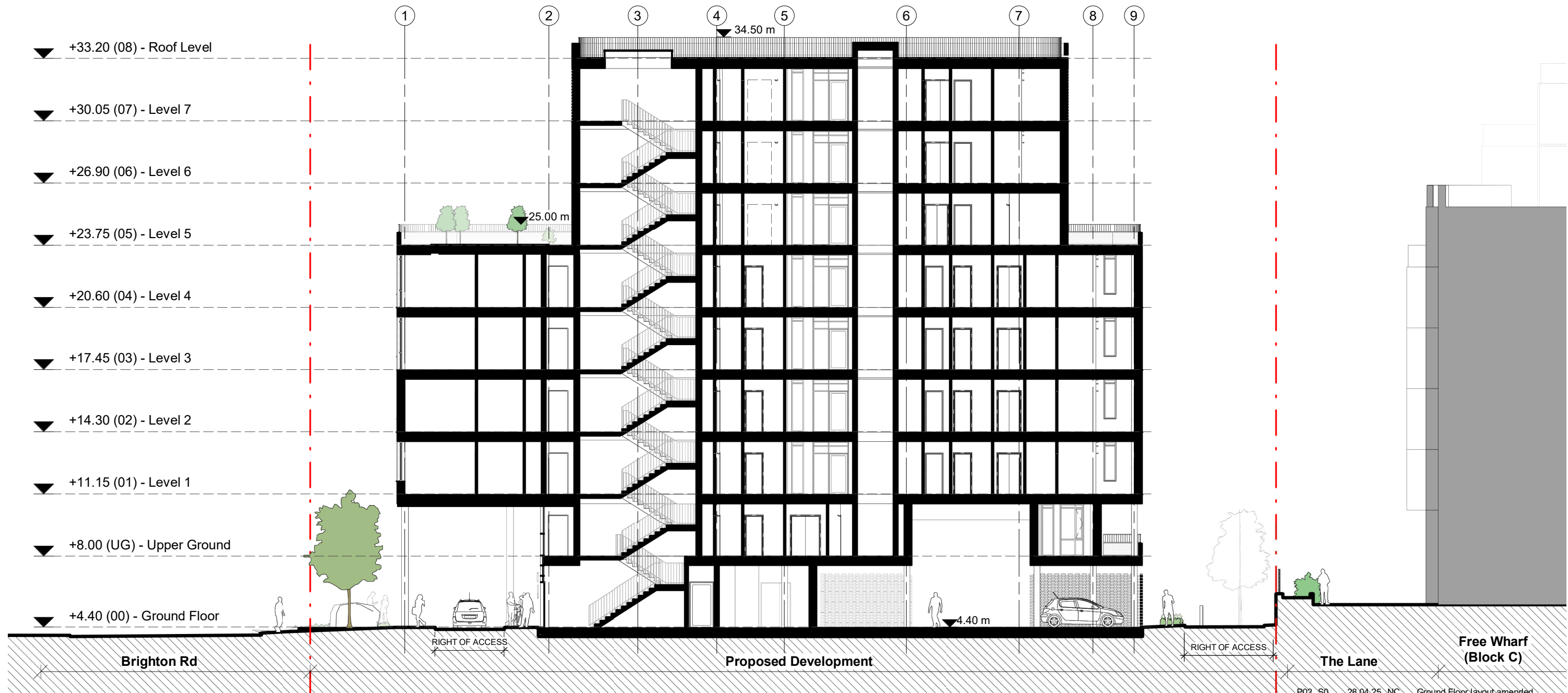
1 Section 01 1 : 200
