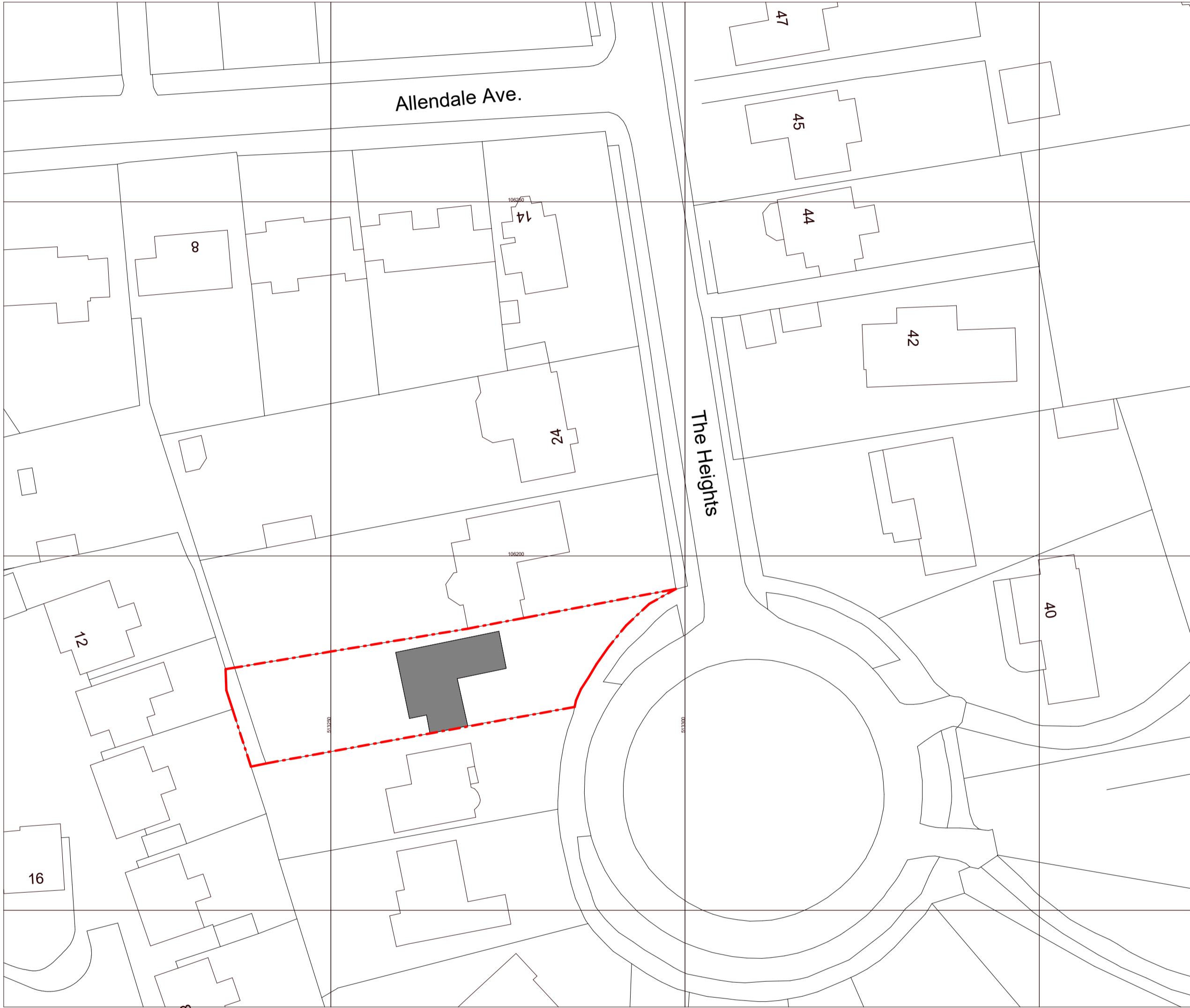
1 Block Plan 1 : 500
