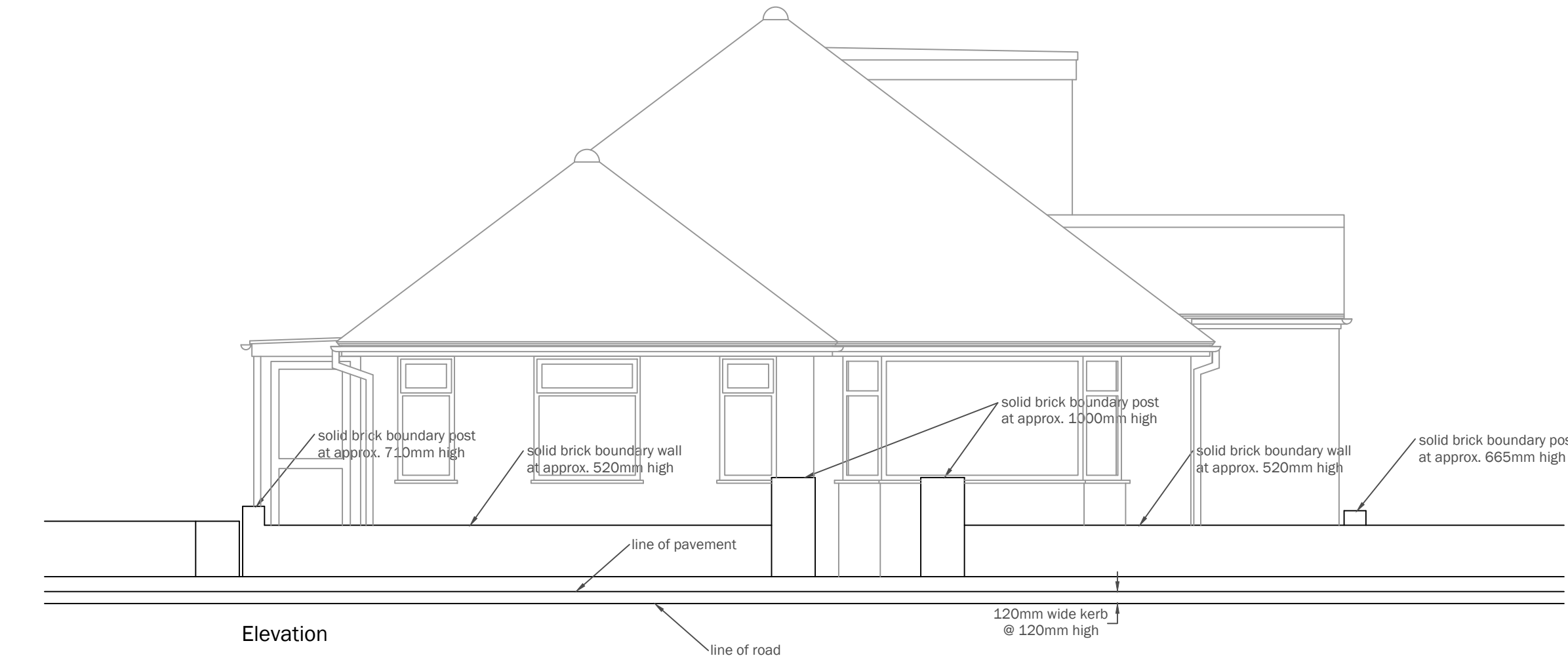
Elevation
