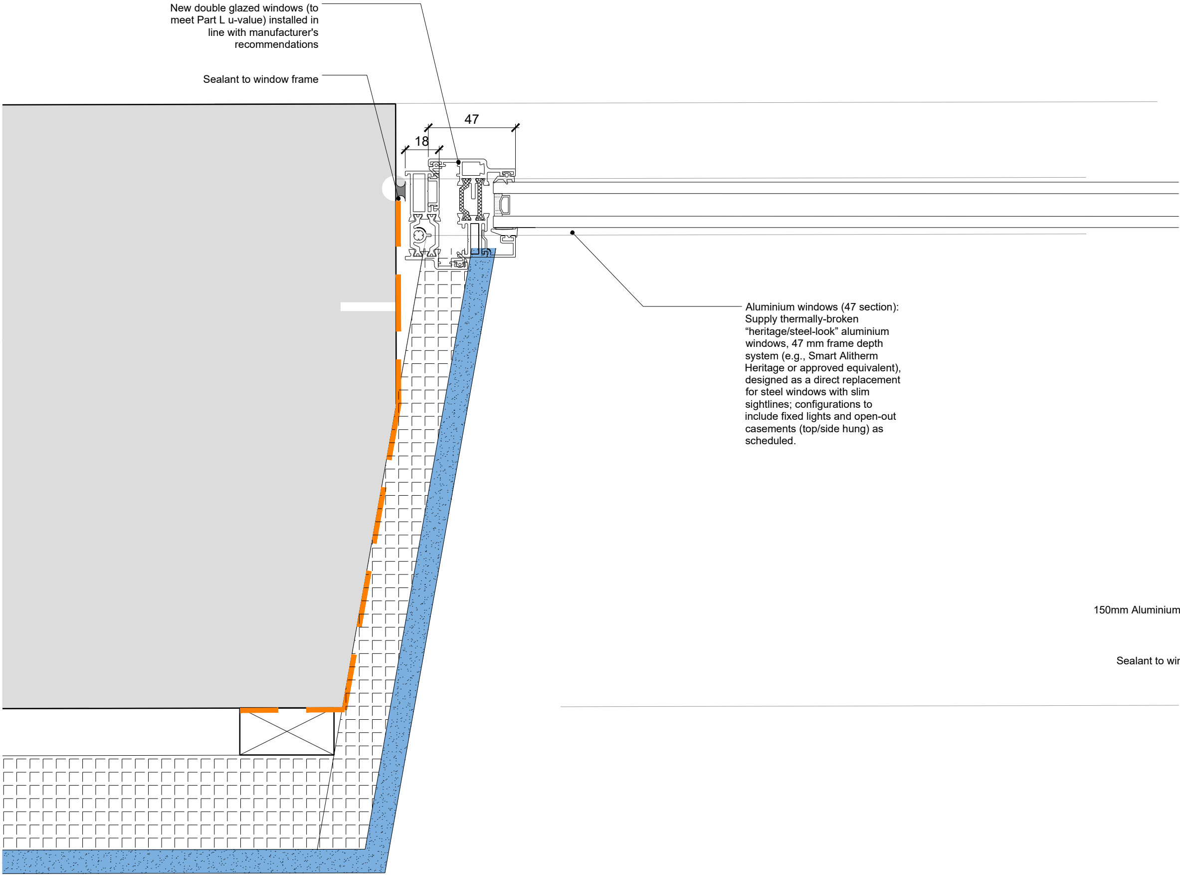
Window Jamb Detail 1:2
