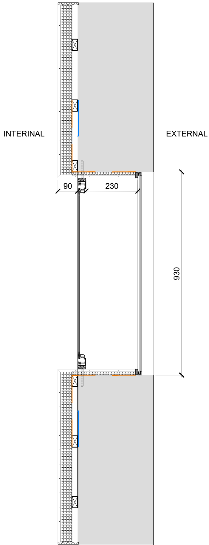
F1 - EW6 Window Section 1:10
