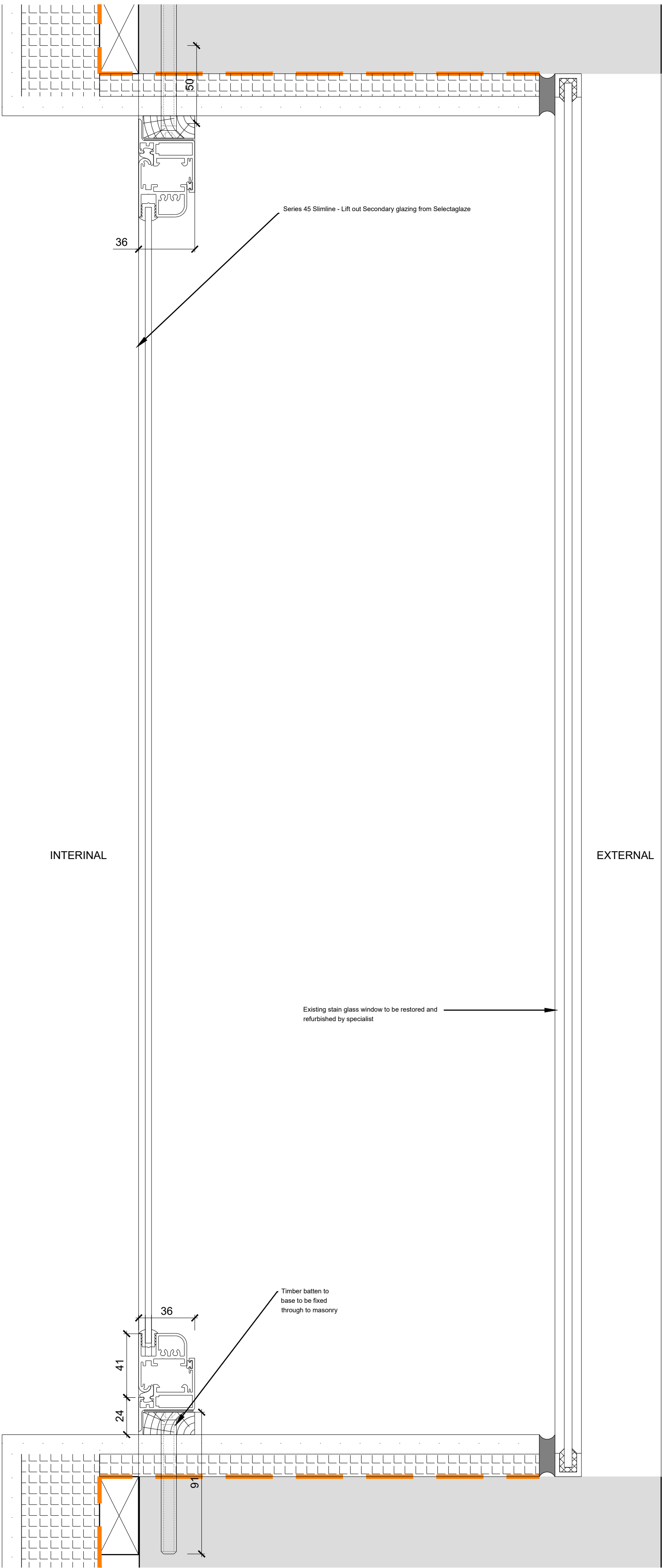
F1 - EW6 Window(Cill/Head) Detail 1:2
