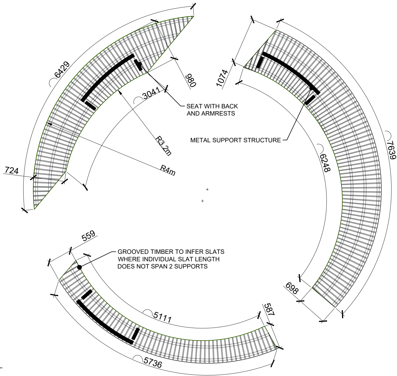
3 PLAN 1:50
