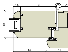
Jamb Section
