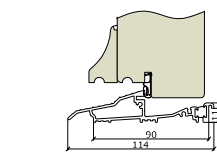
Jamb Section
