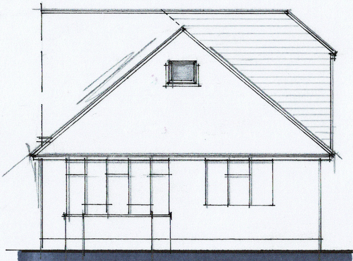
SIDE (w)
